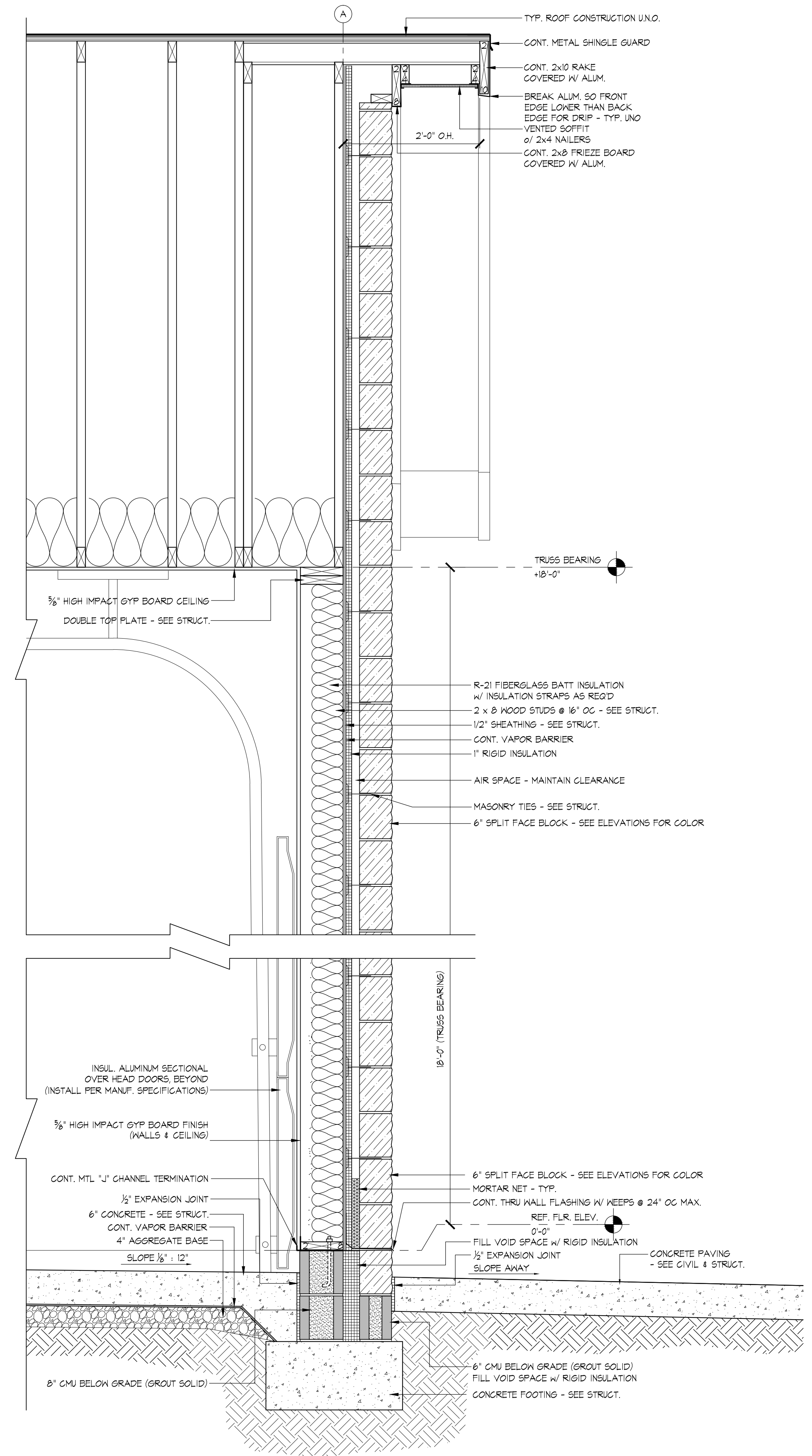
1 WALL SECTION SCALE: 1"=1'-0"
