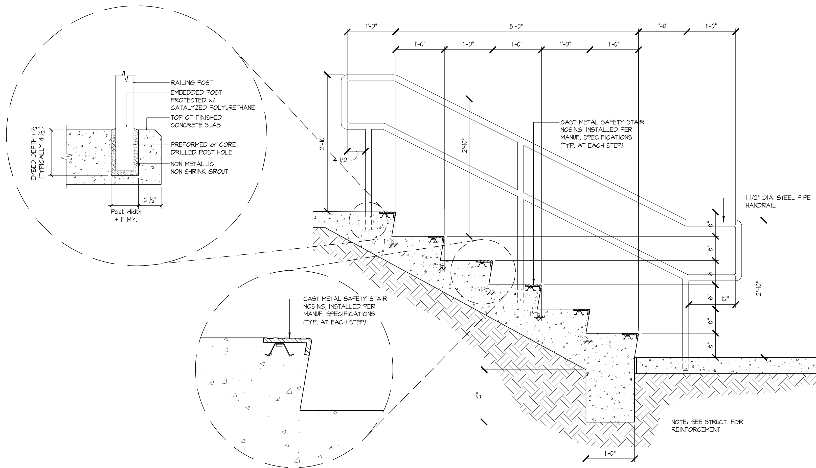
2 CONC. STAIR DETAIL SCALE: 1"=1'-0"
